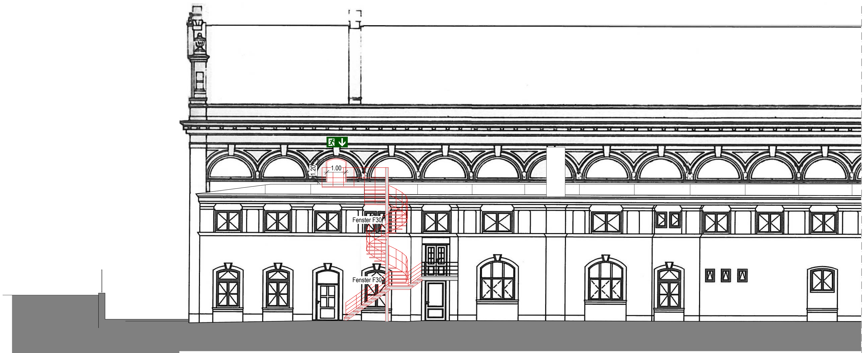
Ansicht Nord
