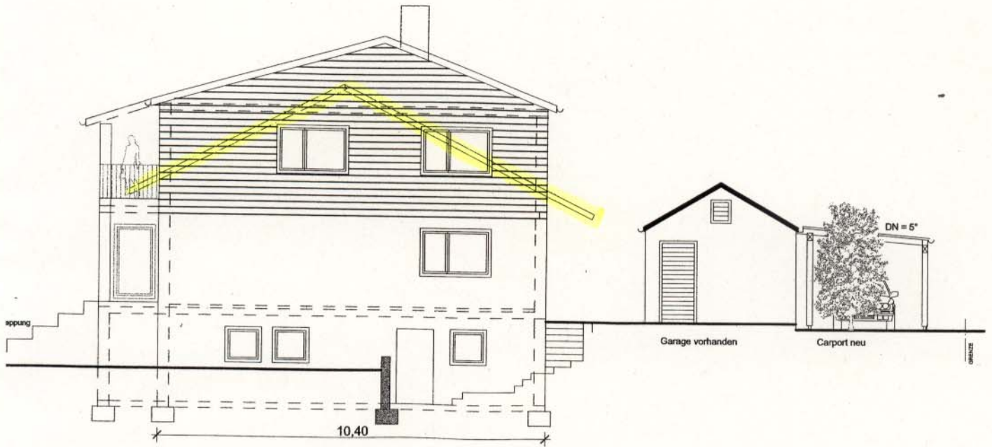
ANSICHT OST
