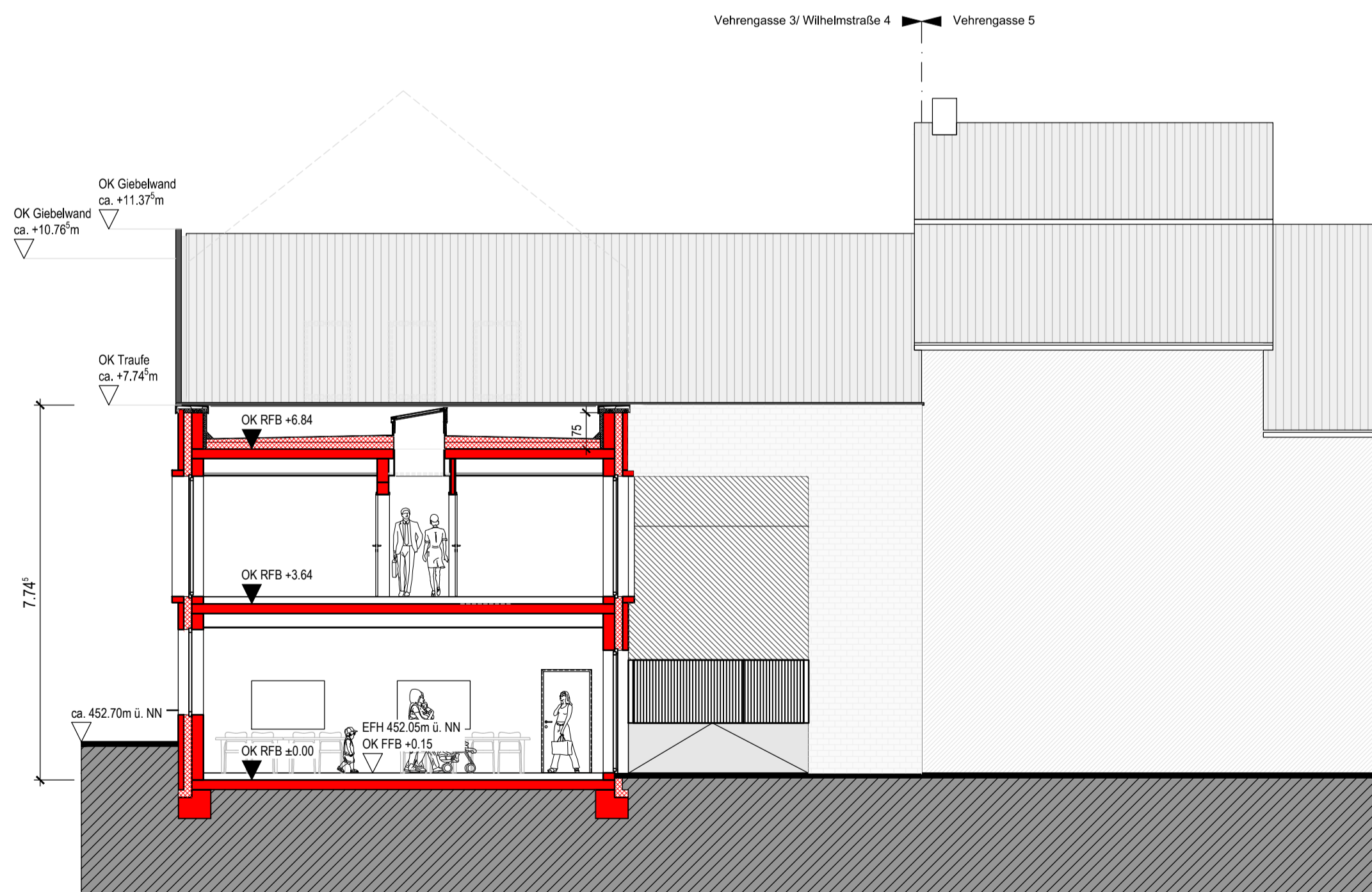
SCHNITT S03
