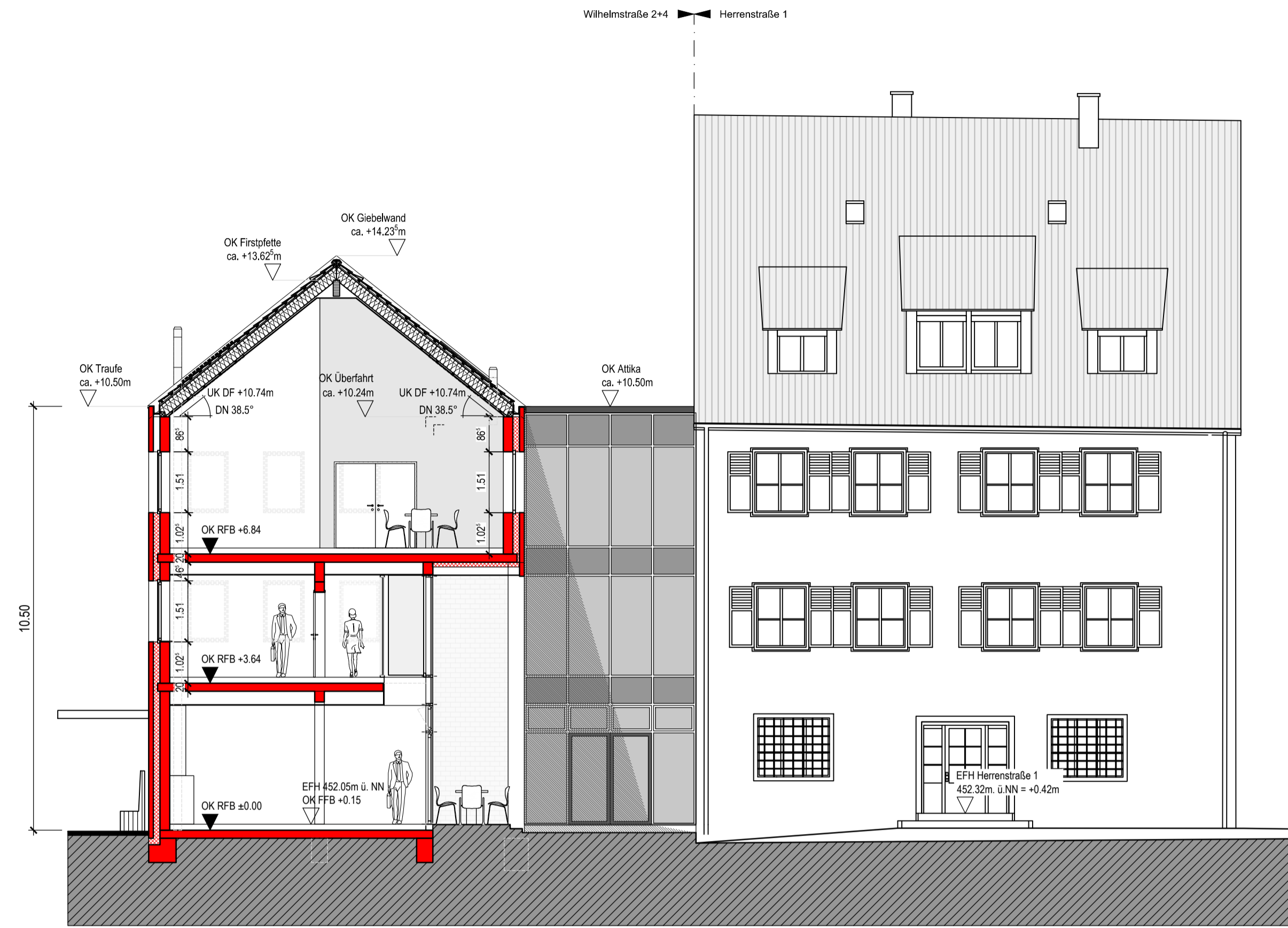
SCHNITT S01
