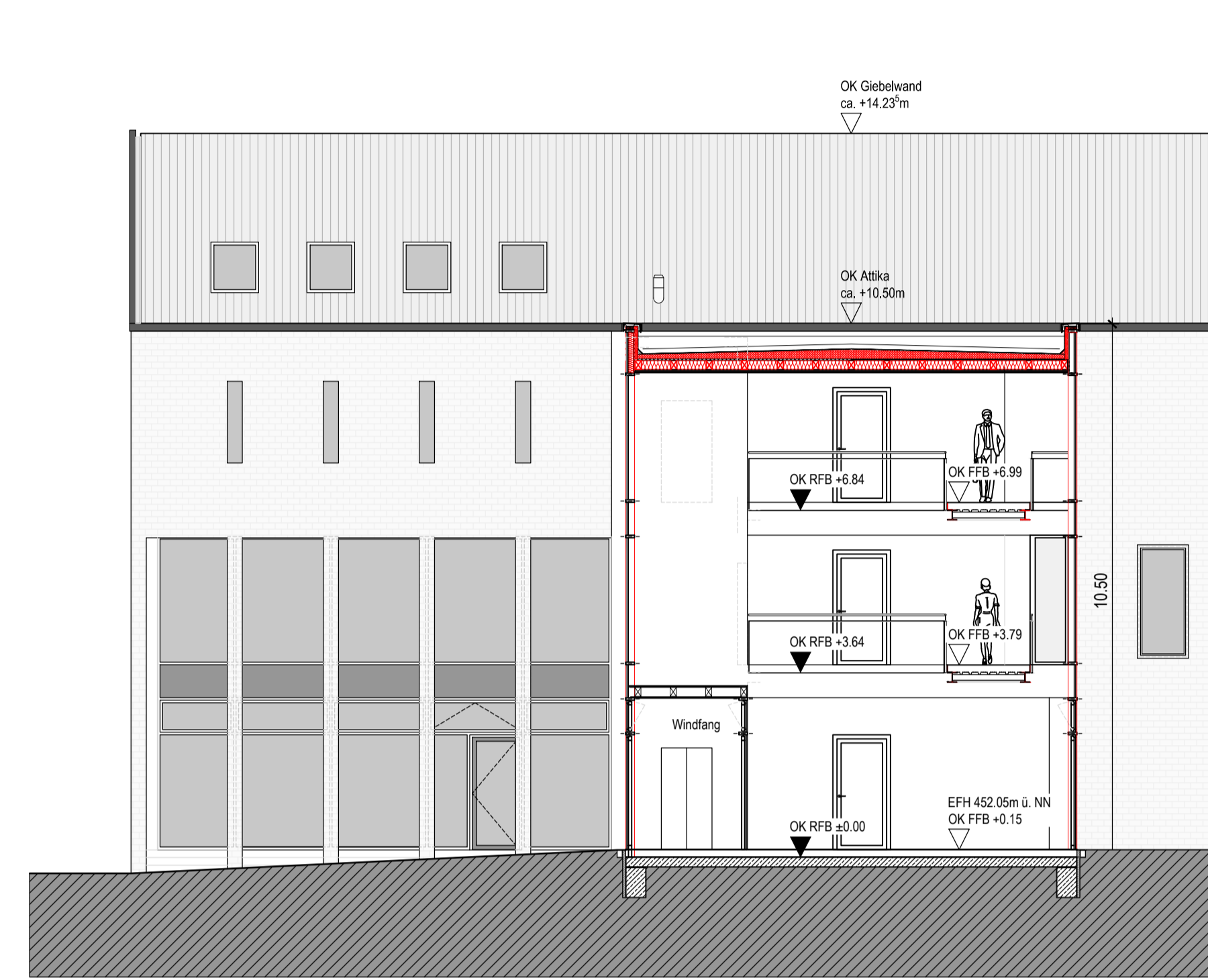
SCHNITT S02
