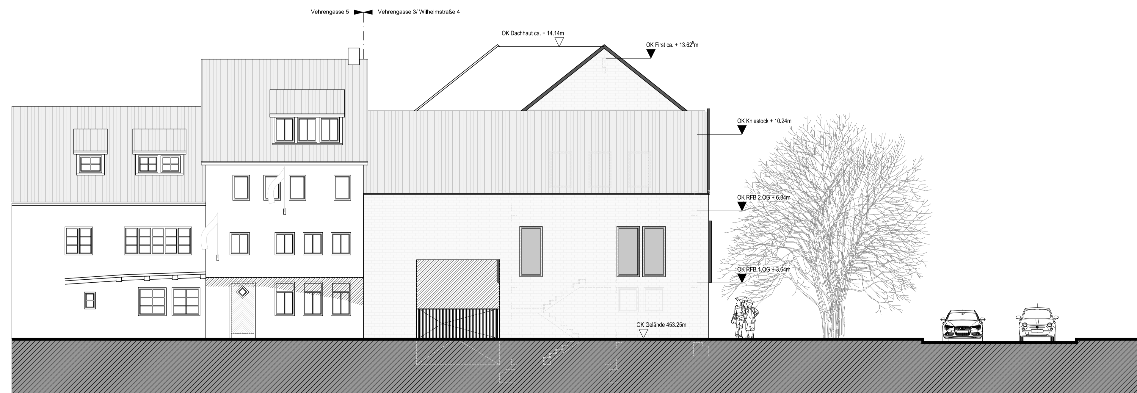
OSTANSICHT
