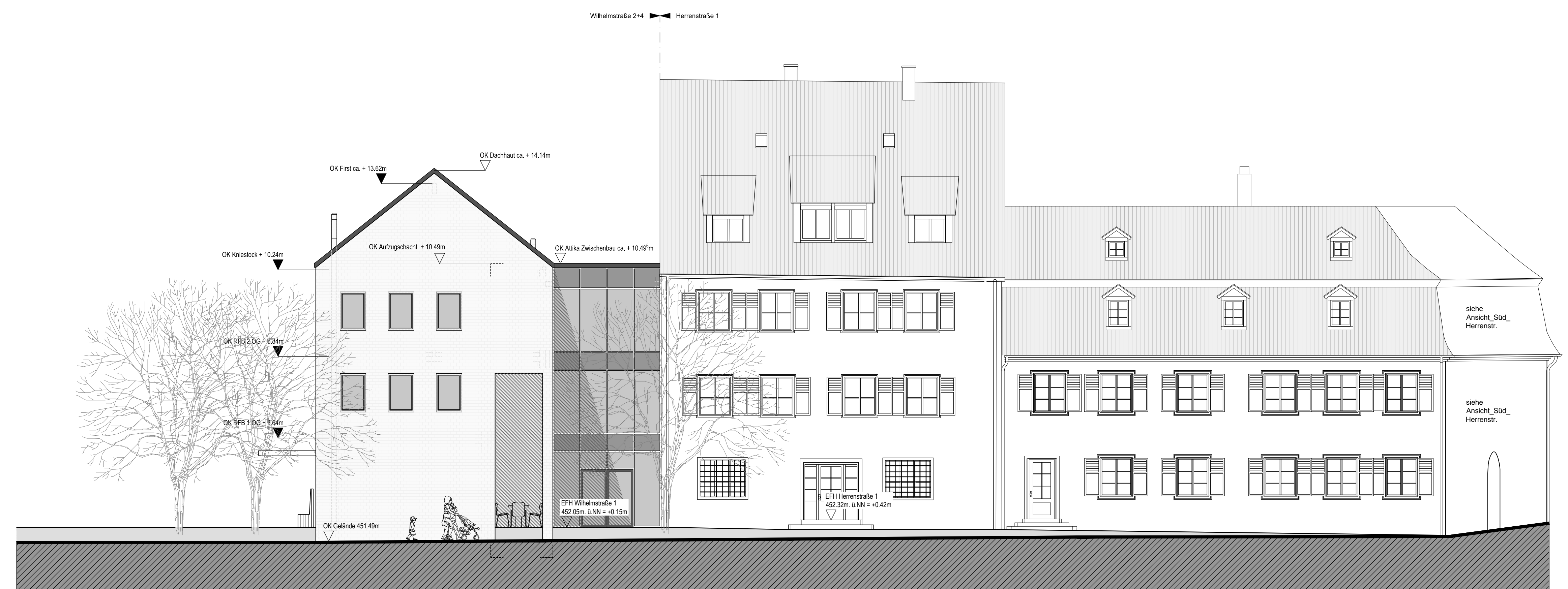
WESTANSICHT
