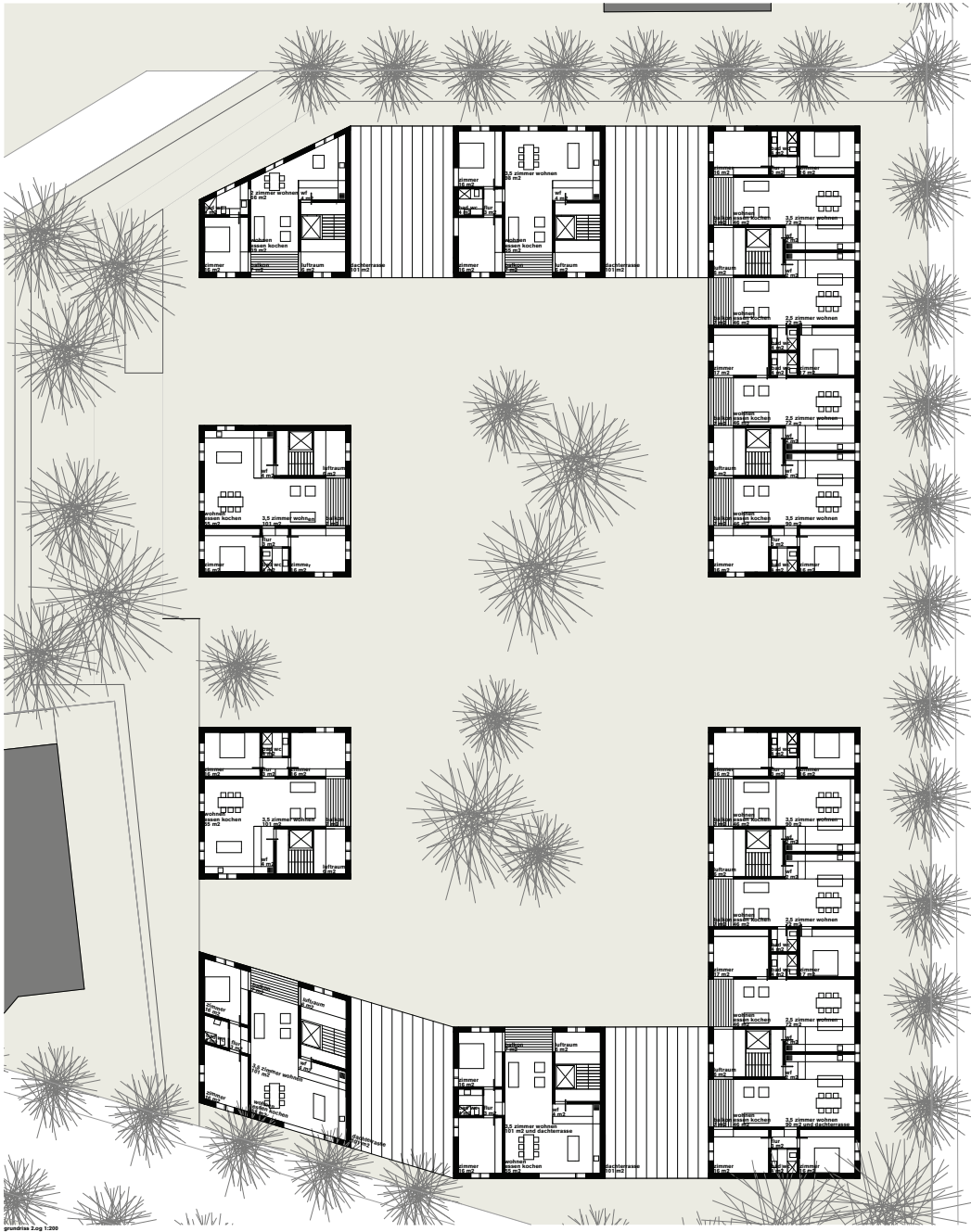
maßstab 1:200
