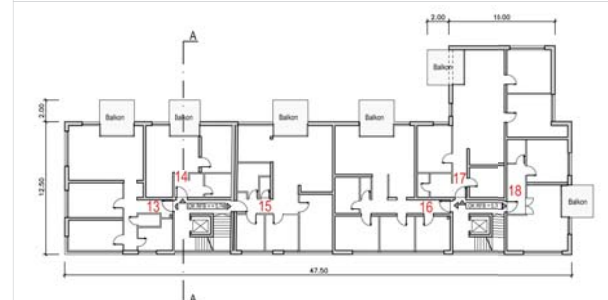
Grundriss 2. Obergeschoss
