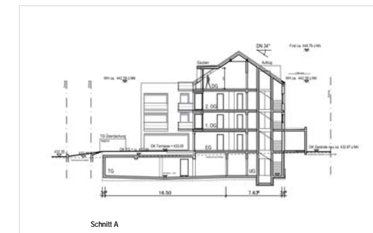
Schnitt A
