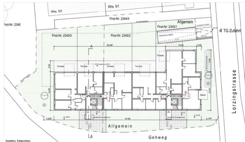
Grundriss Erdgeschoss
