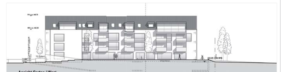
Ansicht Garten / West
