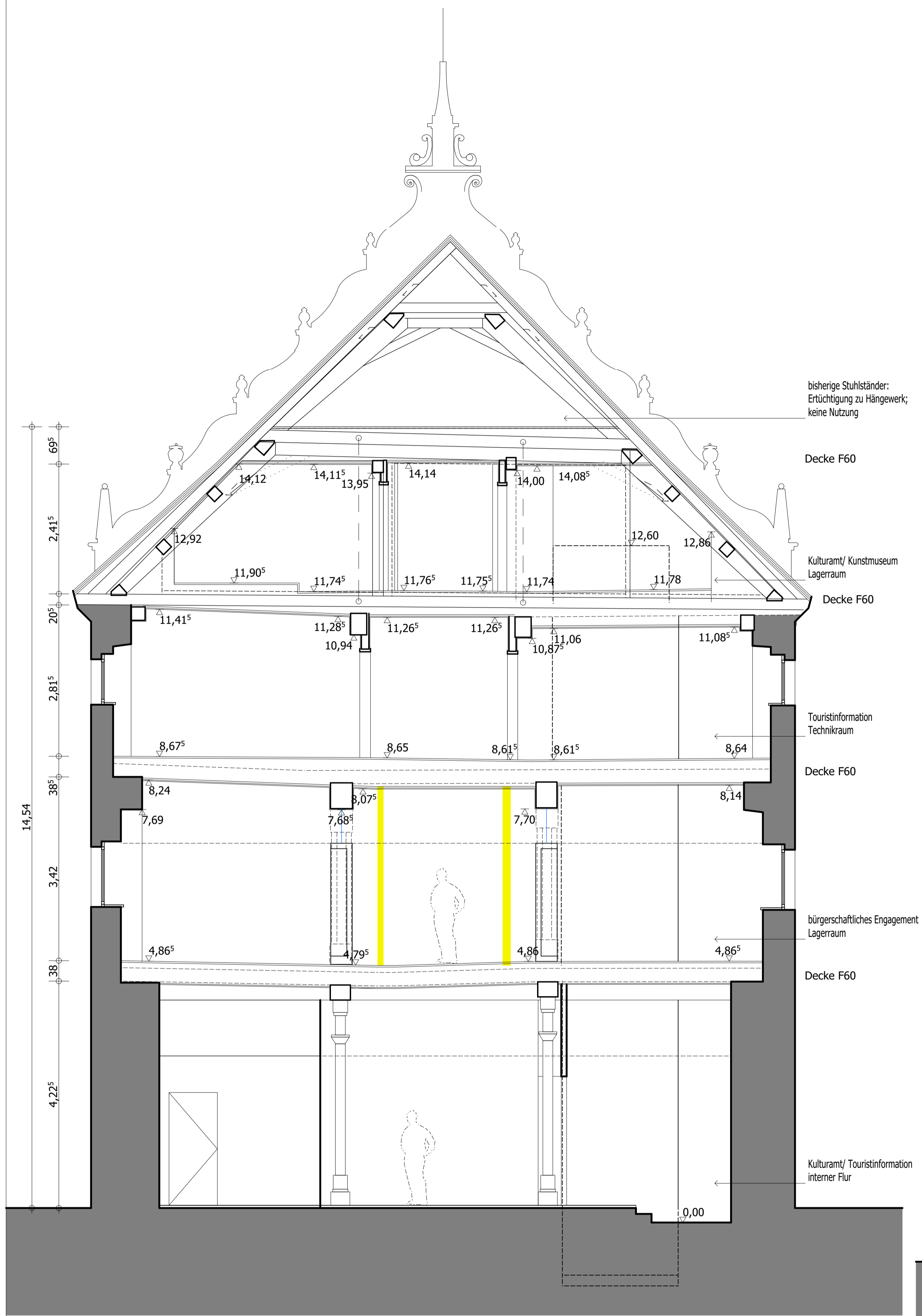
Querschnitt 1
