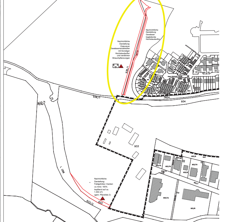
Übersichtsplan externer Ausgleichsmaßnahmen M 1:2.500
