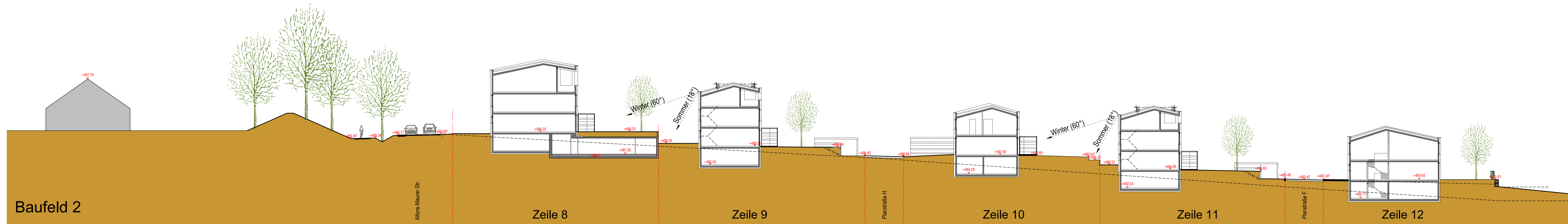
Schnitt Baufeld 2
