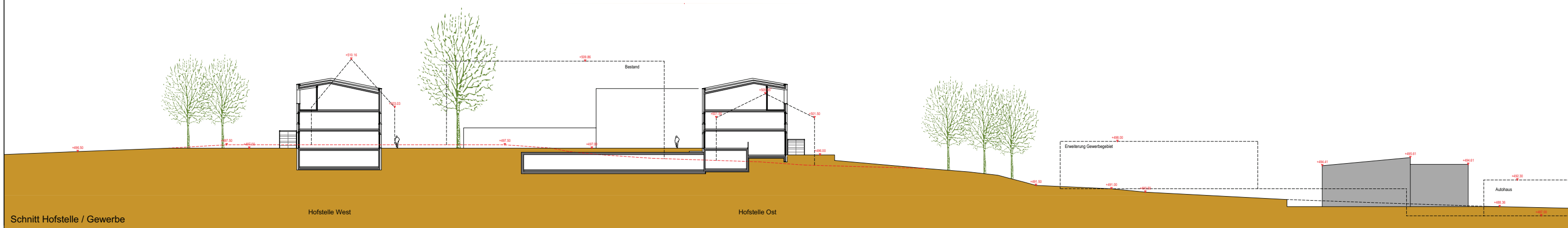
Schnitt Baufeld 1
