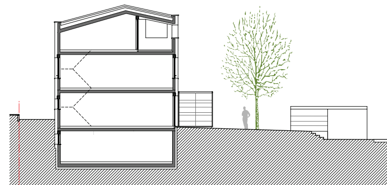
Schnitt
