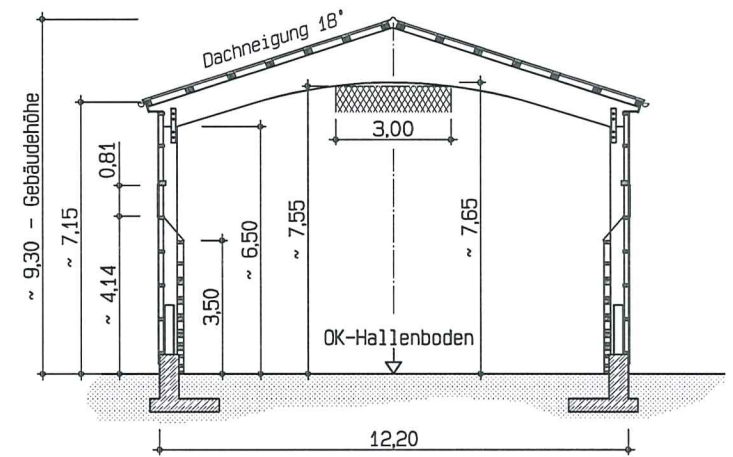
Hallenschnitt, sk=1.5
