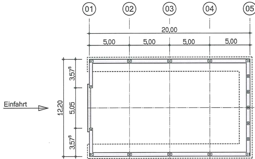
Grundriss Hallenfundament
