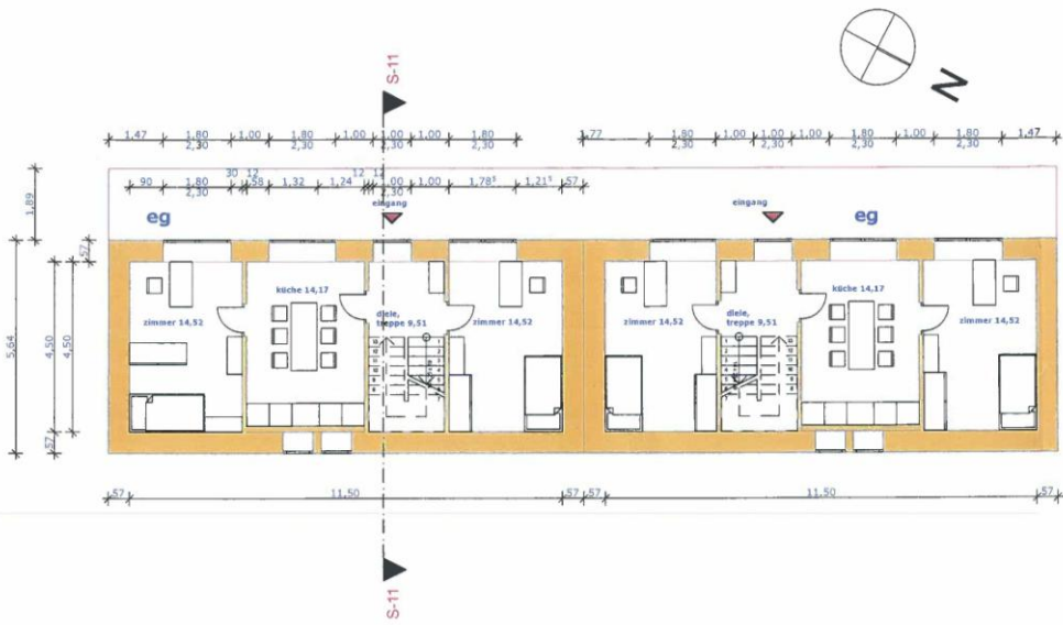
grundriss EG M 1:100
