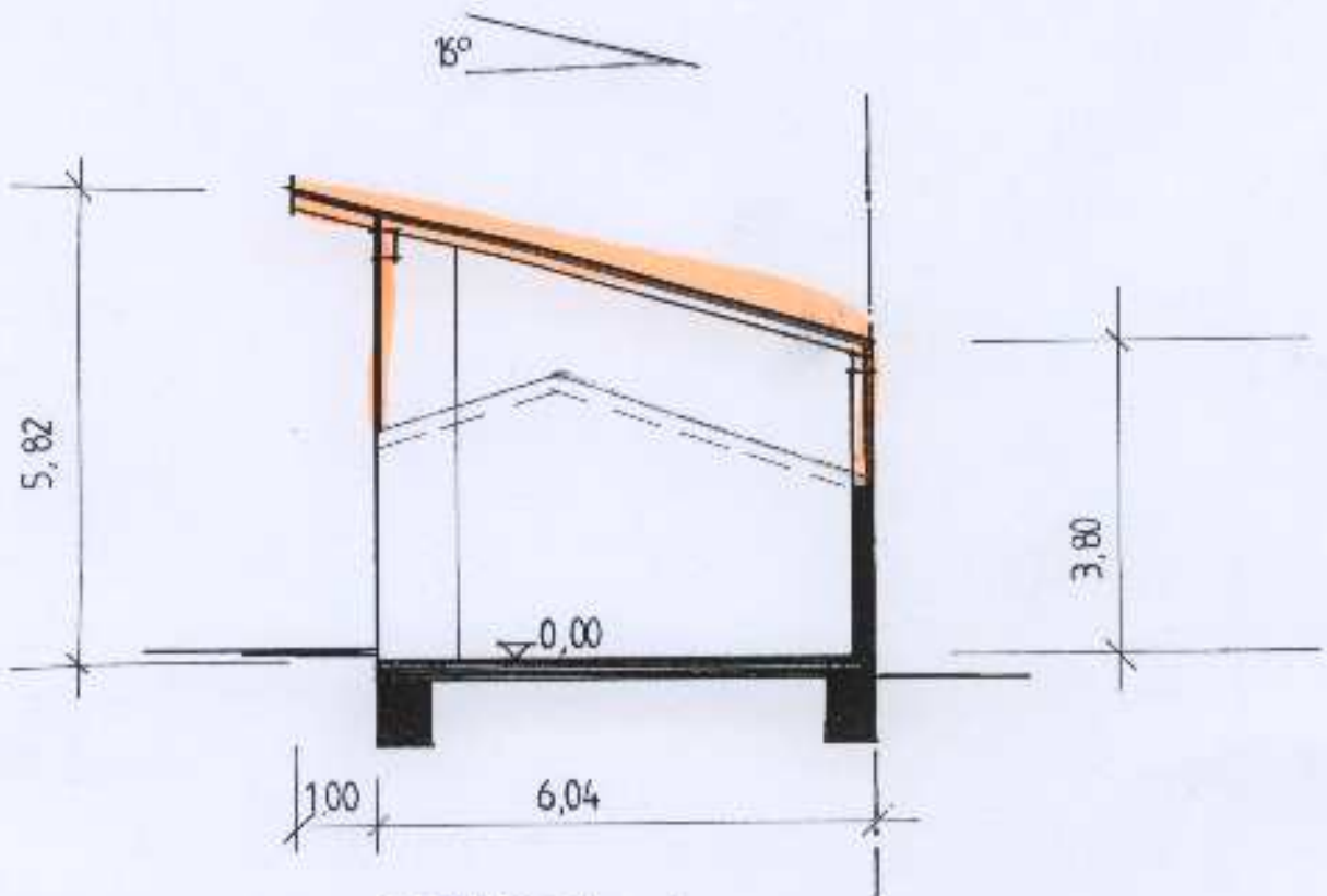
SCHNITTA - A
