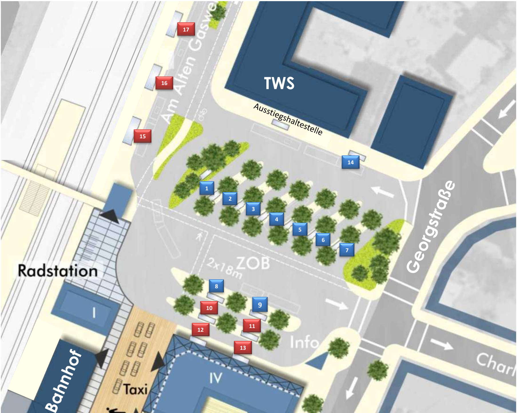
Erweiterung ZOB in Ravensburg
