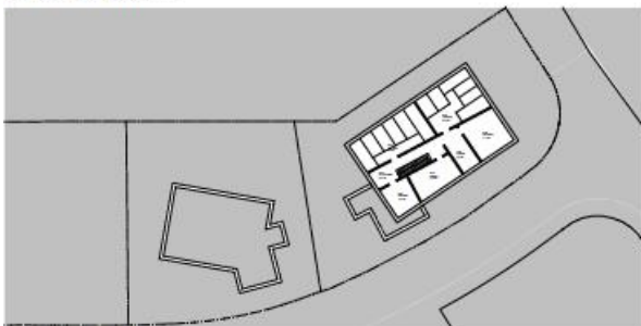
Untergeschoss M 1:200
