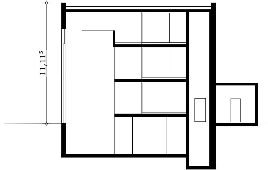
Schnitt 2
