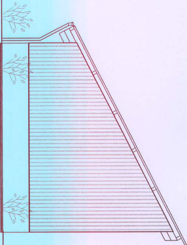
Ansicht Ost M 1:100
