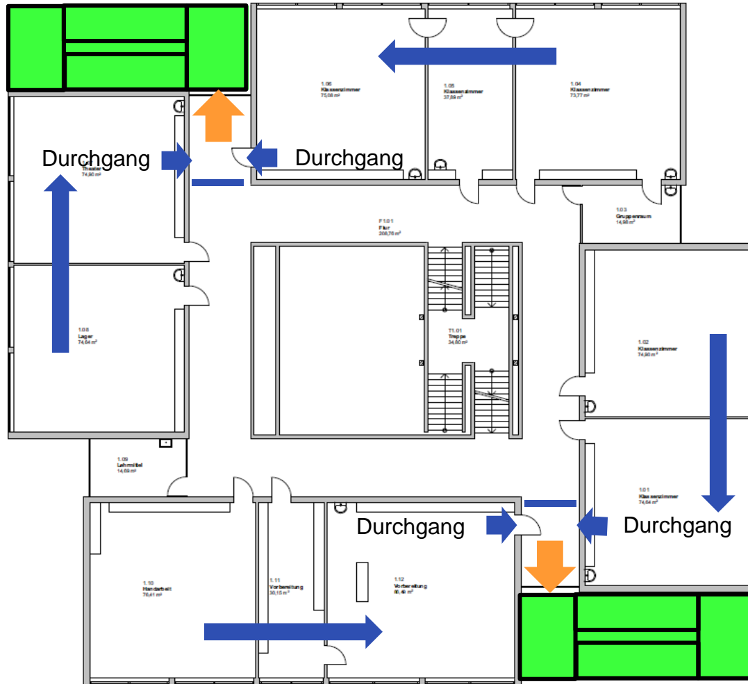
Fluchttreppenhaus 2
