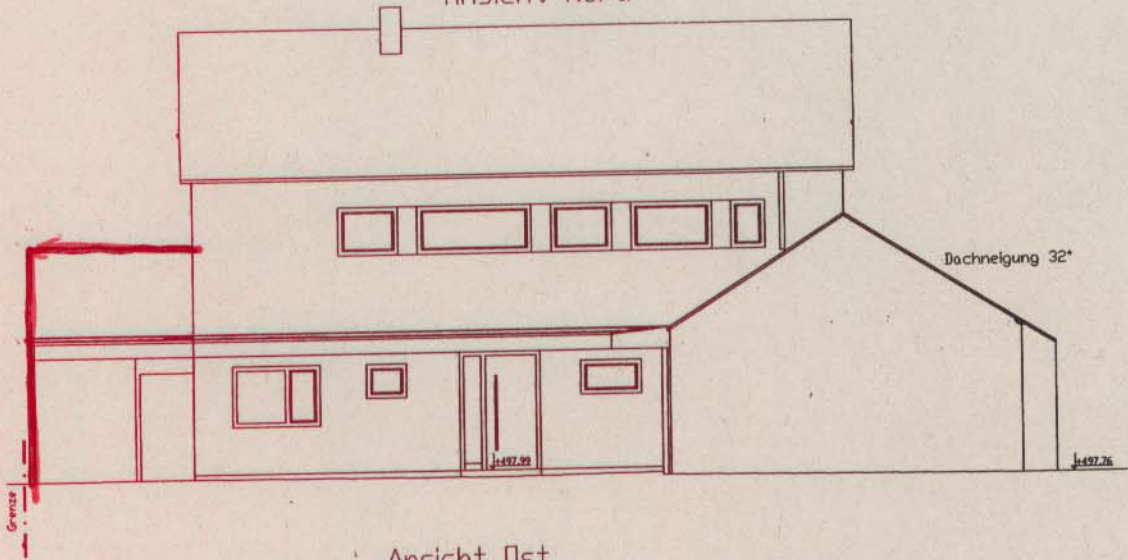
Ansicht Ost
