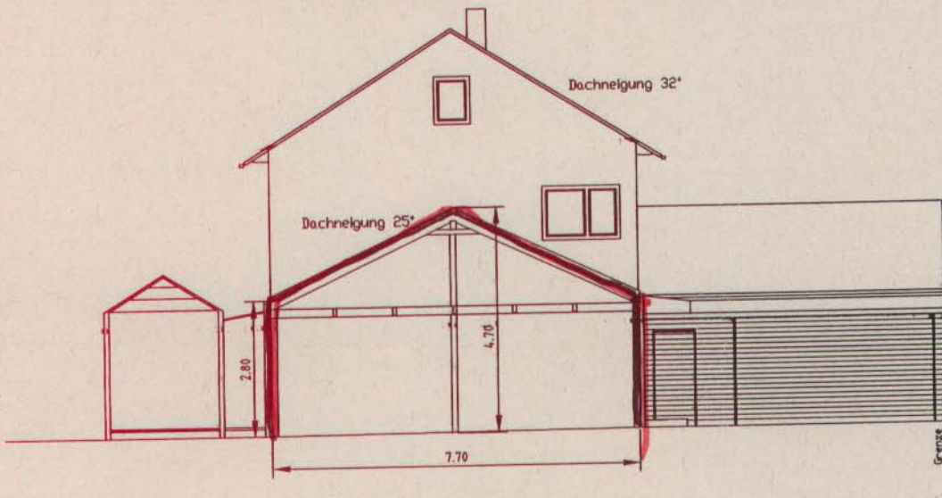
Ansicht Süd
