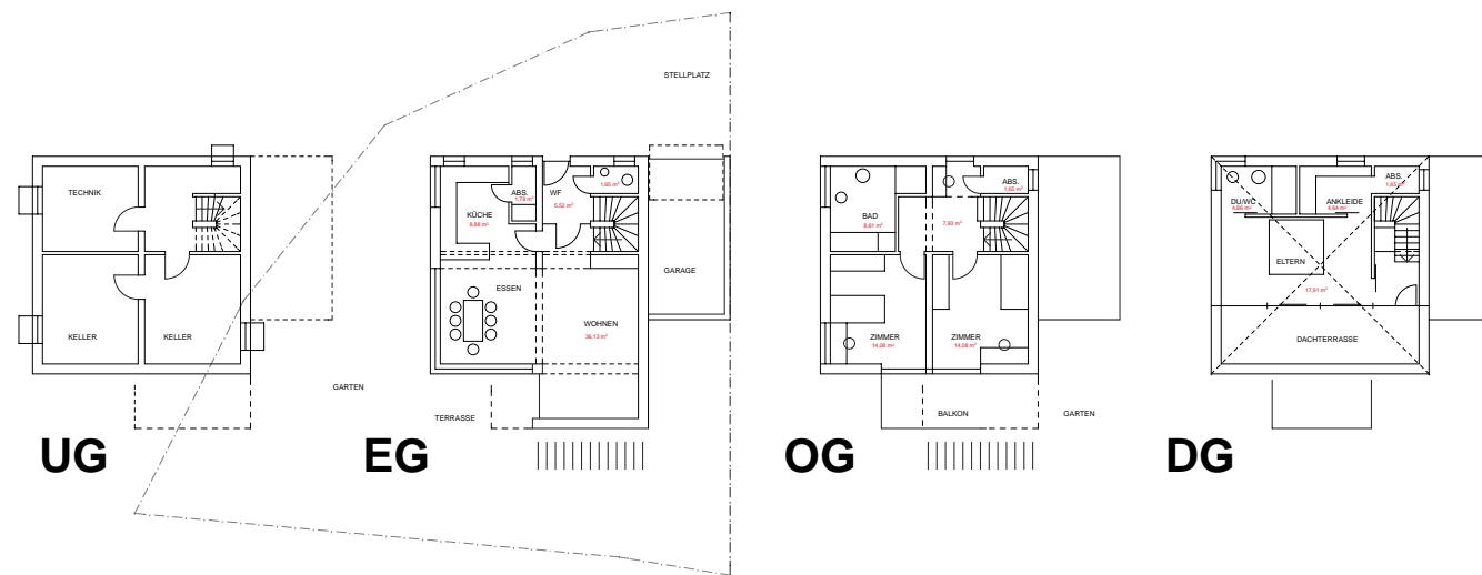
GRUNDRISSE EINFAMILIENHAUS
