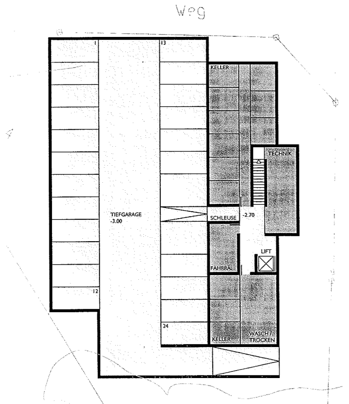
Grundriss Untergeschoss
