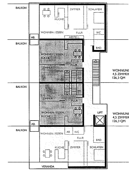
Grundriss Alternative 2 - Maisonette 1. OG
