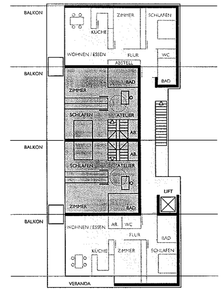
Grundriss Alternative 2 - Maisonette 2. OG
