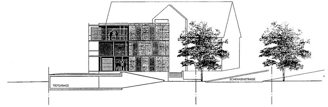
Ansicht Süd-Ost
