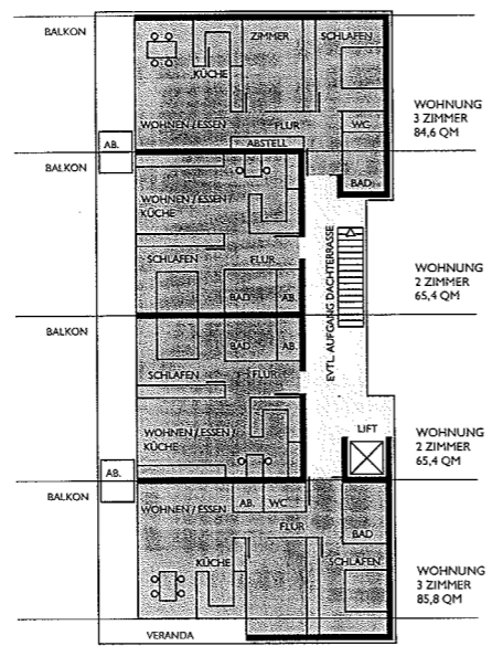
Regelgrundriss EG und OG
